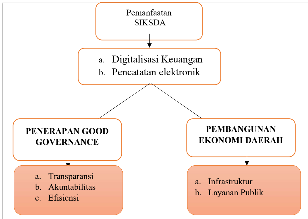
Gambar 1 Kerangka Konseptual
