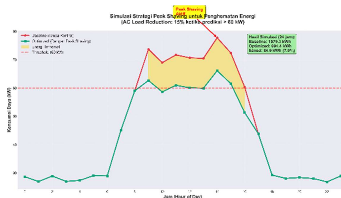
GAMBAR 8: Simulasi Penghematan Energi Menggunakan Strategi Peak Shaving
