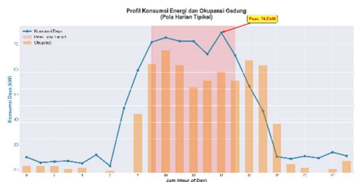
GAMBAR 6: Grafik Profil Konsumsi Energi dan Okupansi Gedung
